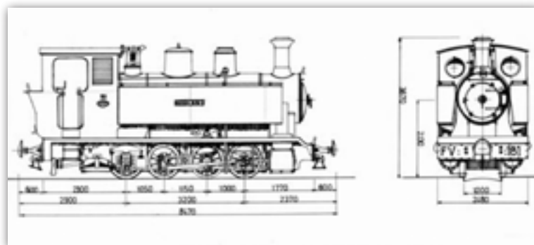
Placencia lokomotoraren modelua, Couillet 030 T motakoa.
